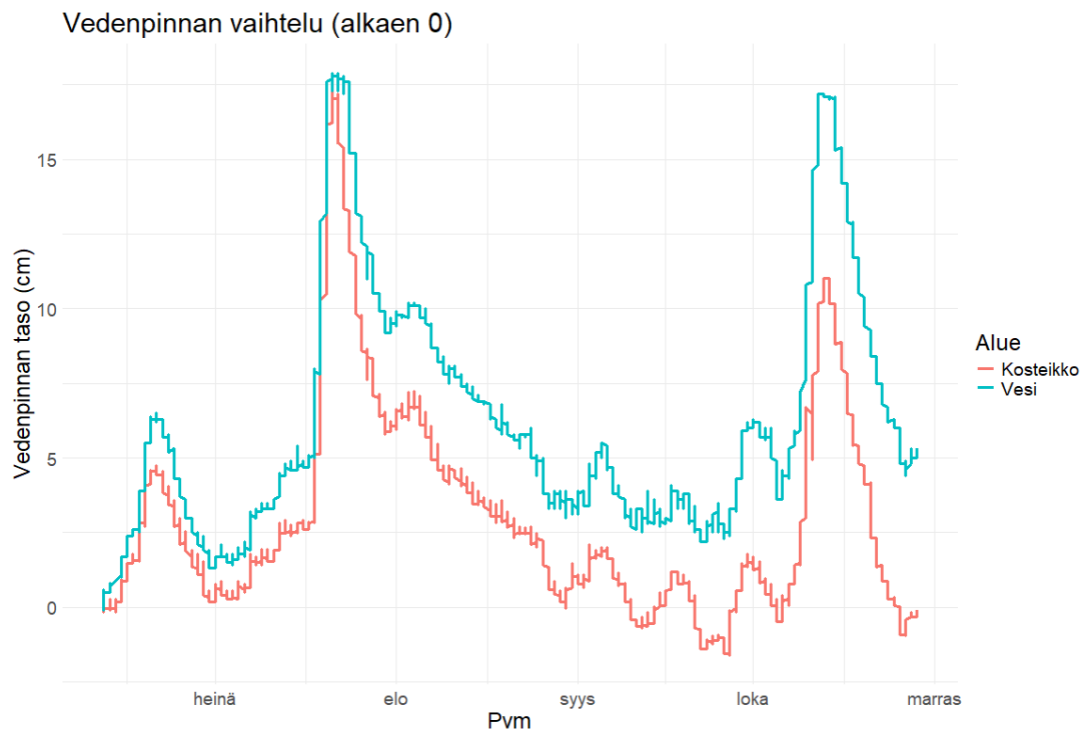
Kuva 14. Vedenpinnan tason vaihtelu Kurunnevan avovesialueella kasvukaudella 2024. Lähtötilanteen 0-taso on se hetki, kun loggerit on asetettu alueelle mittausten aloitushetkellä. Loggerit mittasivat tästä tapahtunutta muutosta vedenpinnan tasossa.
