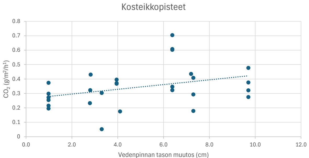
Kuva 19. CO 2 vapautumisen suhde vedenpinnan tason muutokseen Kurunnevan kosteikolla.
