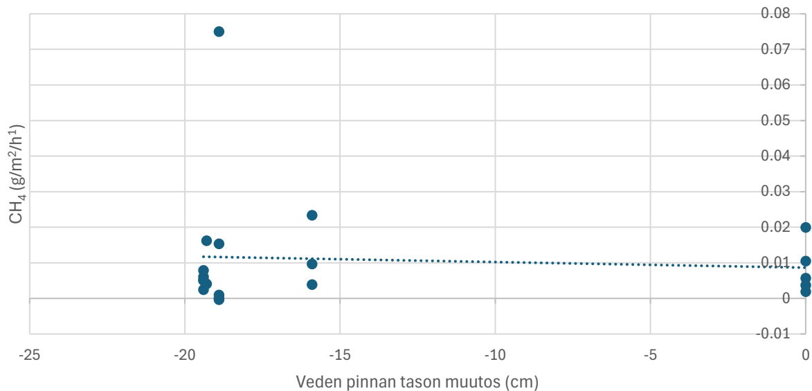
Kuva 10. CH 4 -vuon suhde veden pinnan tason muutokseen Karjonevan avovedessä.
