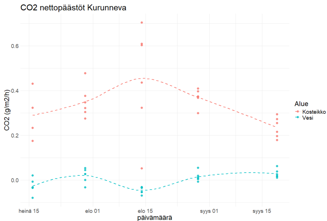
Kuva 17. Hiilidioksidin nettopäästöt Kurunnevalla kosteikolta ja avovedestä mitattuna kasvukaudella 2024.
