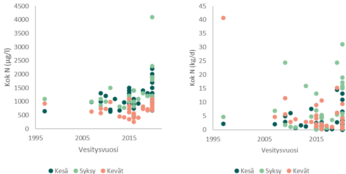
Kuva 6. Kosteikoilta lähtevän veden kokonaistypen (Kok N) pitoisuus ( \mu\text{g/l} ) ja hetkellinen kuorma ( \text{kg/d} ) kesän, syksyn ja kevään näytteenottokierroksilla suhteutettuna alueen vesitysvuoteen.
