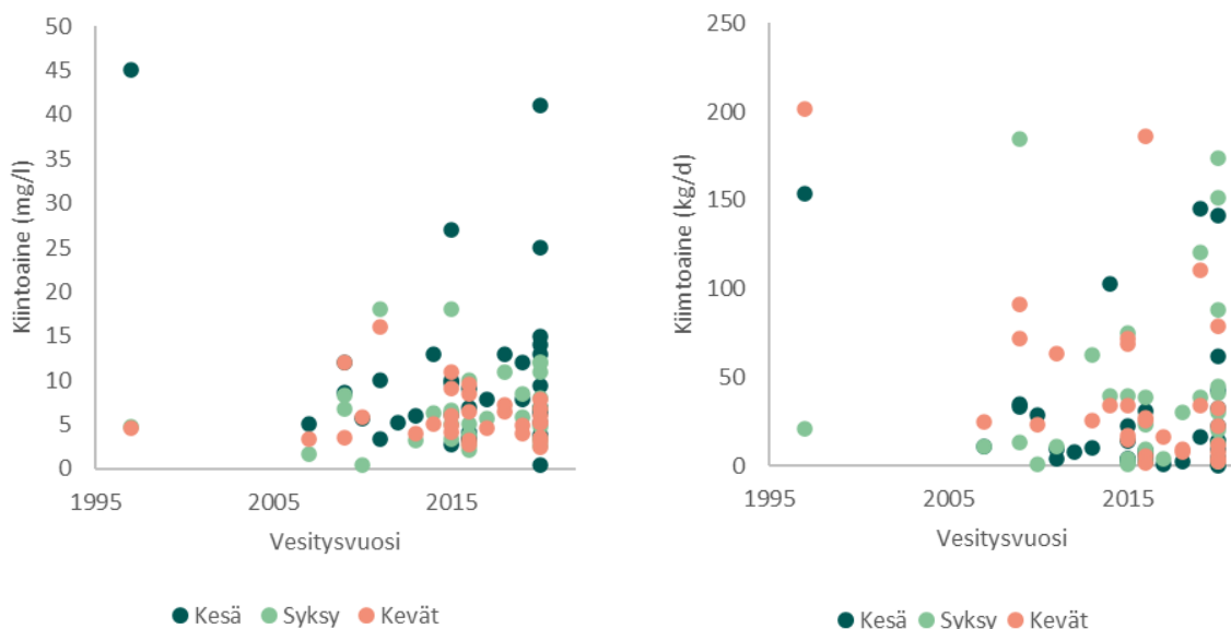
Kuva 14. Kosteikoilta lähtevän veden kiintoaineen (GF/C) pitoisuus (mg/l) ja hetkellinen kuorma (kg/d) kesän, syksyn ja kevään näytteenottokerroksilla suhteutettuna alueen vesitysvuoteen.
